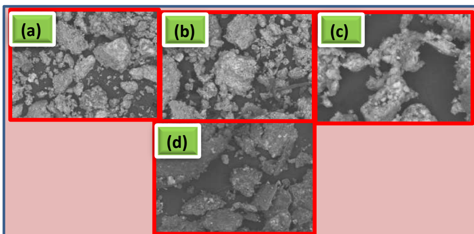
Fig.2: SEM images of ZnO/VB 1 /PVC NCs
